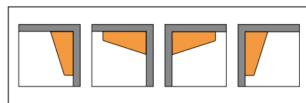
Możliwości zabudowy Schlüter-SHELF-E-S3
