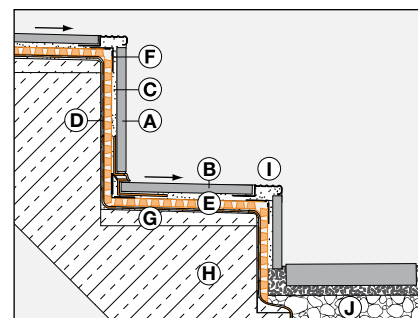
Schody zewnętrzne z drenażem zespolonym Schlüter®-DITRA-DRAIN 8
